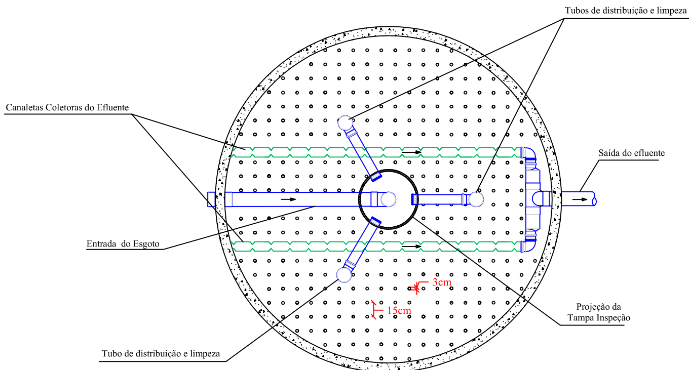
Planta Baixa
