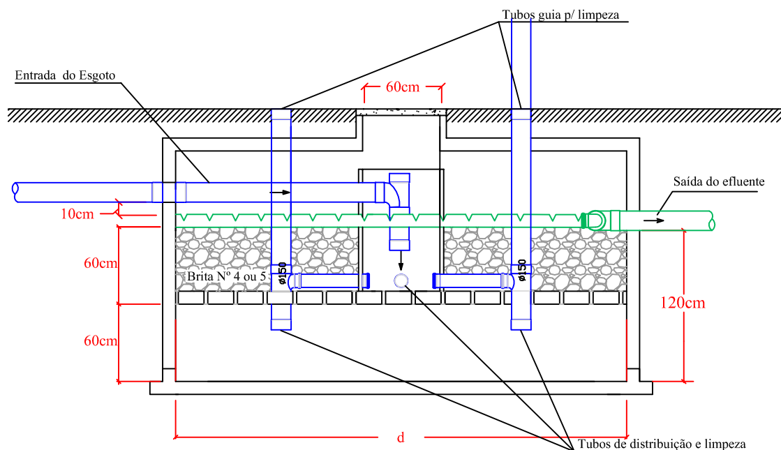
Corte
