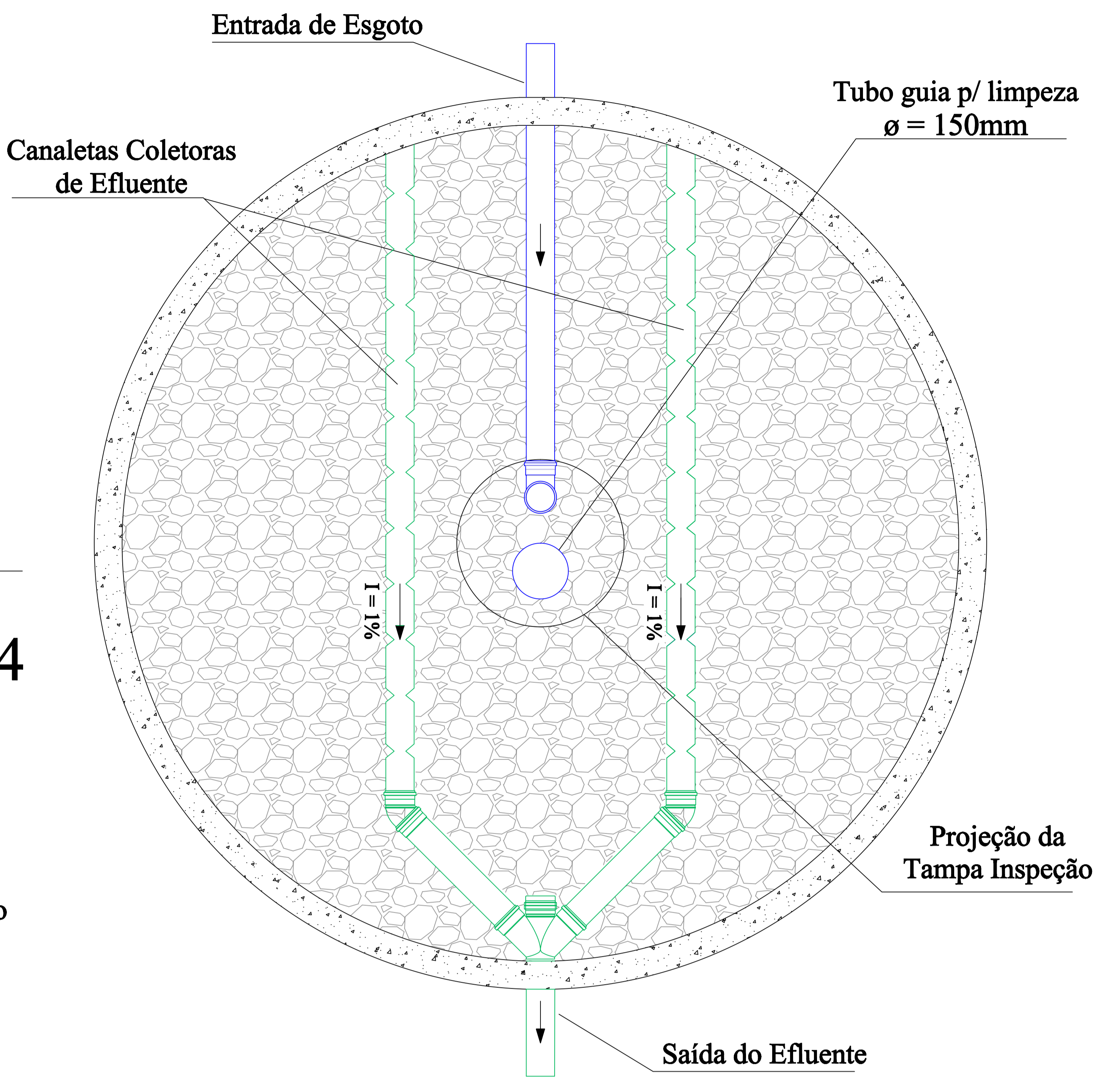
Planta Baixa 2 - 2
