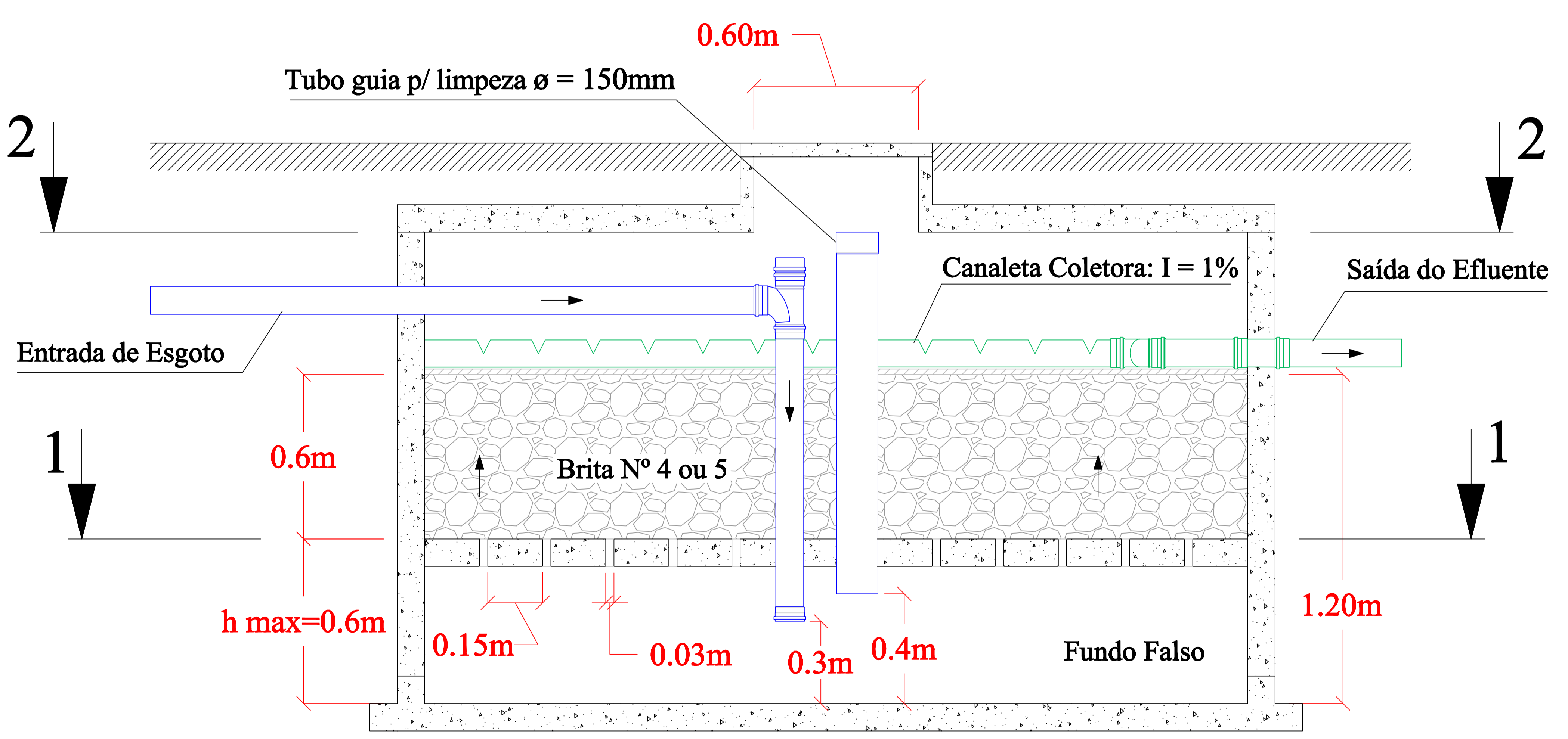
Corte 3 - 3
