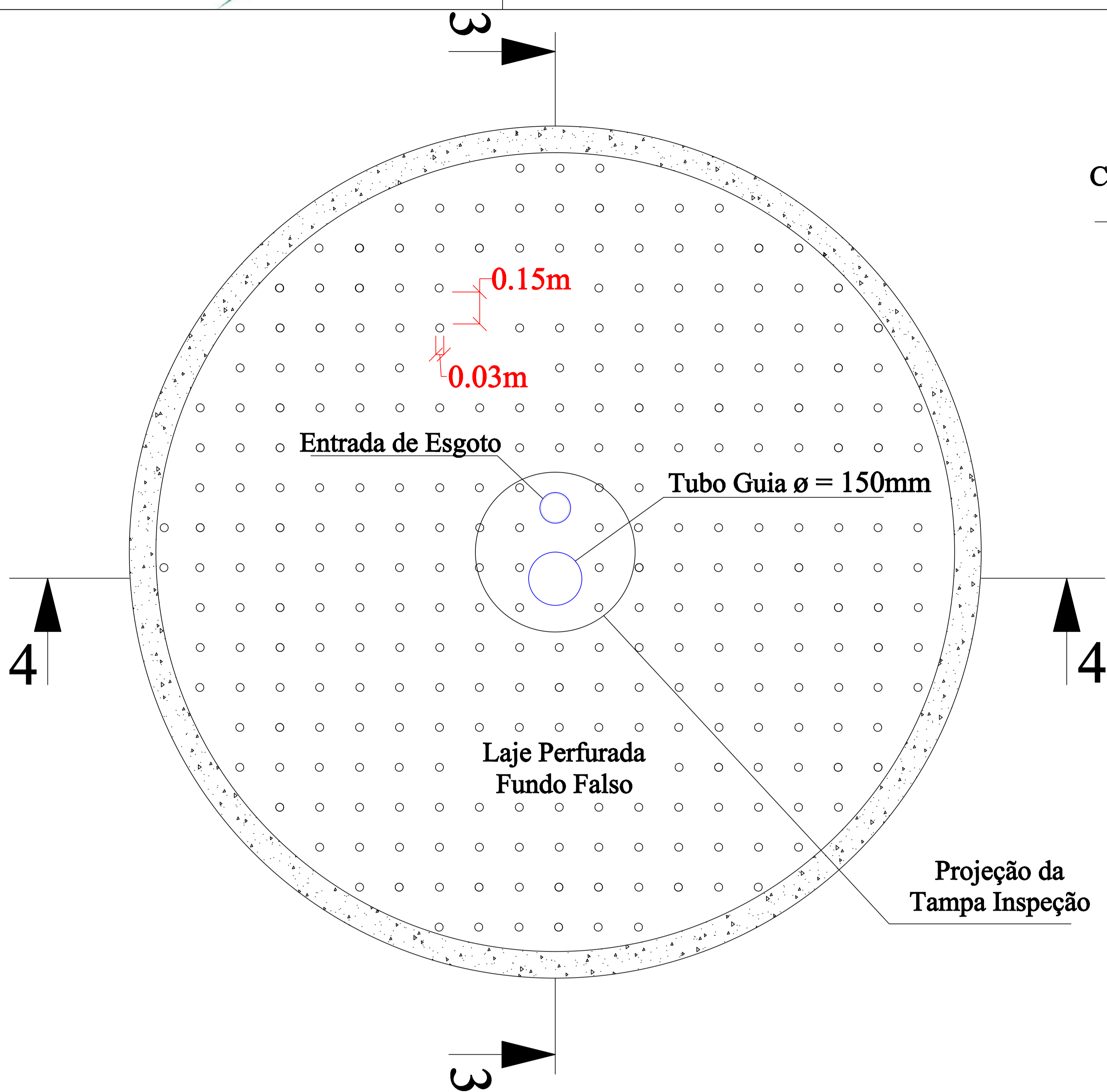
Planta Baixa 1 - 1
