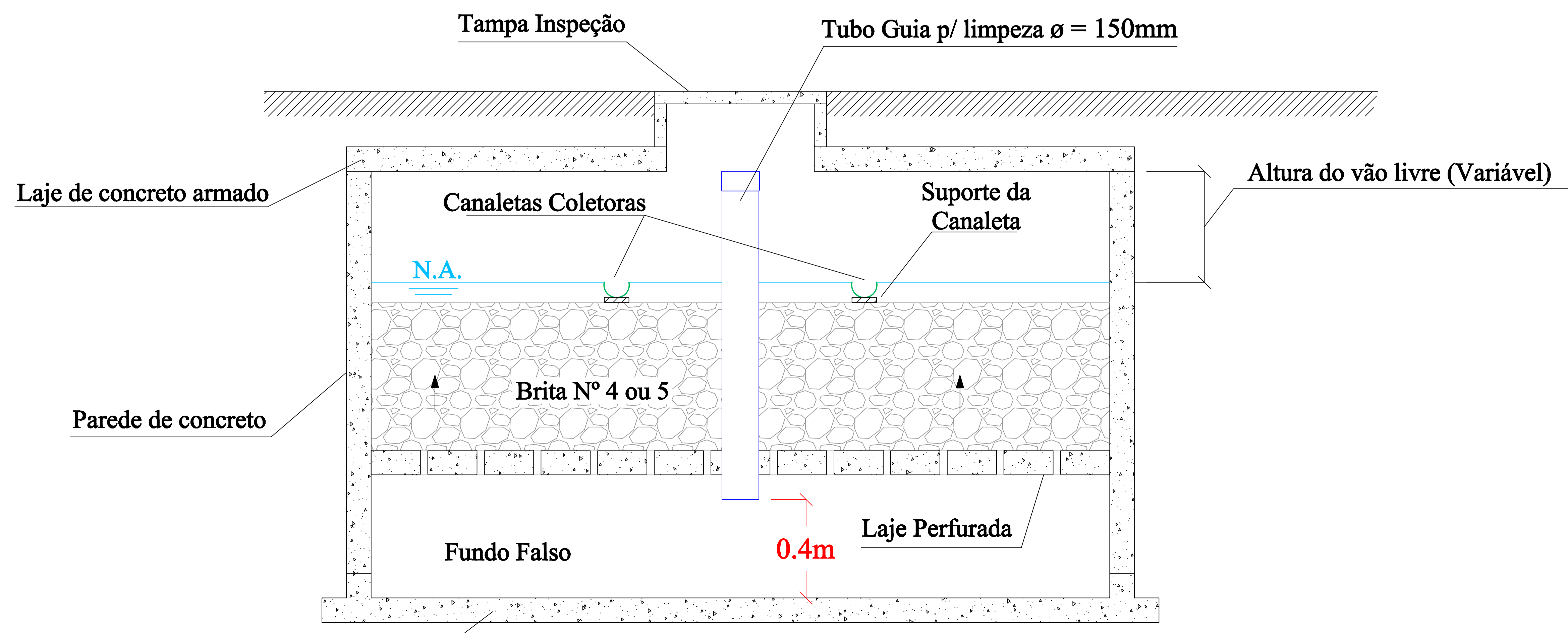
Corte 4 - 4
